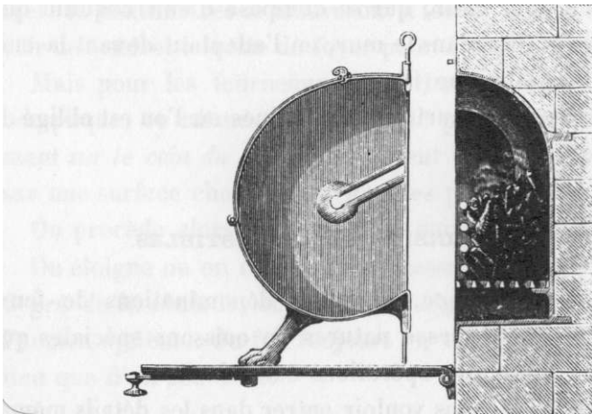
Fig. 17. Coupe du fourneau modèle montrant l'appareil pour rôtir.
